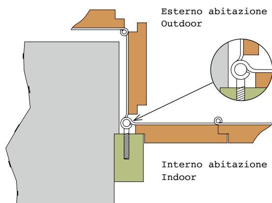
7 Bandella snodata alla mestrina occhio centrale Articulated hinge mestrina style centred eye
