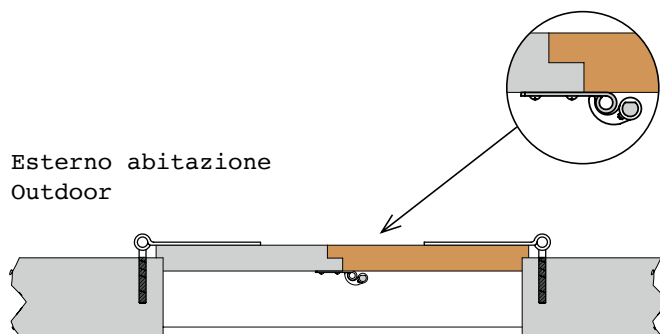
15 Pareggiatore per spagnoletta Alignment bolt for espagnolette
