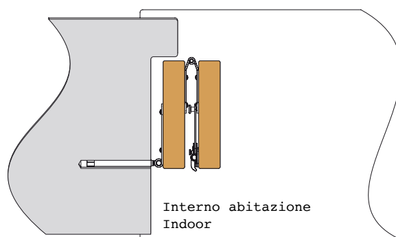
10 Bandella alla vicentina rovescia Reverse Vicenza style hinge
