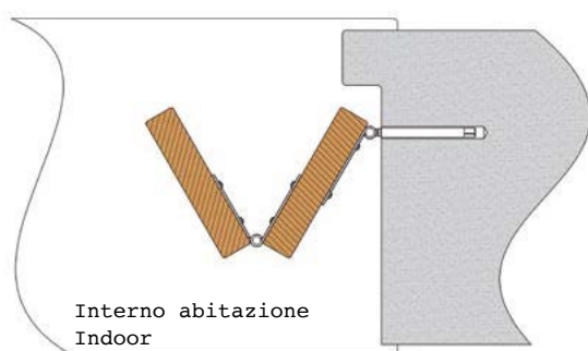
9 Bandella alla vicentina Vicenza style hinge
