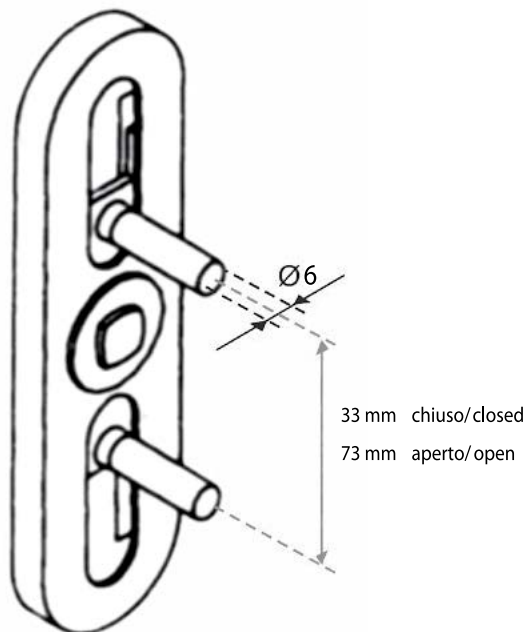
Gioco "gratz" con perni "Gratz" lock with pins
