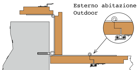
16 Incontro di bloccaggio e allineamento per persiane a libro Securing and aligning junction for building blinds
