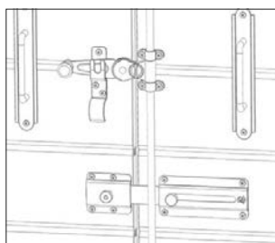
Applicazione sotto la spagnoletta/ Application under espagnolettes
