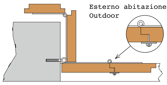
17 Fermo di allineamento a mezzaluna per persiane a libro Aligning stop with screw for folding blinds
