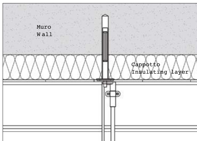
15 Pareggiatore per spagnoletta Alignment bolt for espagnolette
