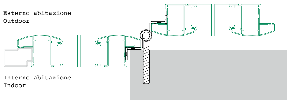
11 Bandella a incasso Embedded hinge
