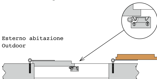
14 Fermo per spranghetta senza battuta Securing stop for espagnolette blinds without rebated edge
